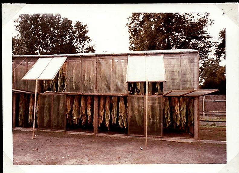
Töves dohányszáritás vasvázas fóliaszátorban.
