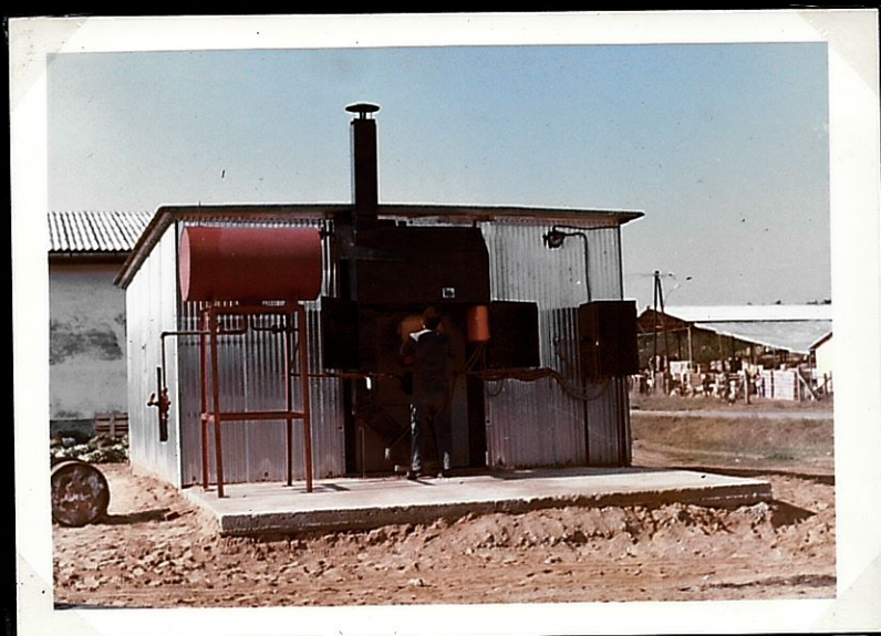
Sirokkó TDO-60 tűsorkeretes szárítóberendezés.
